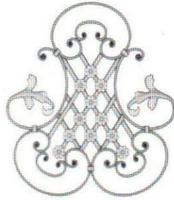
Art. 100-02 (640 x 710mm) 7.000kg 16 x 8mm
