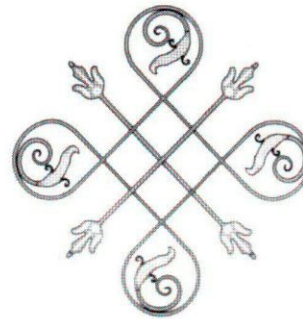
Art. 100-11 (720 x 720mm) 3.500kg 16 x 8mm
