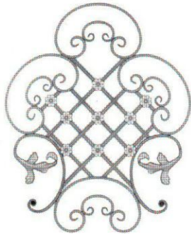
Art. 100-09 (750 x 890mm) 8.500kg 16 x 8mm
